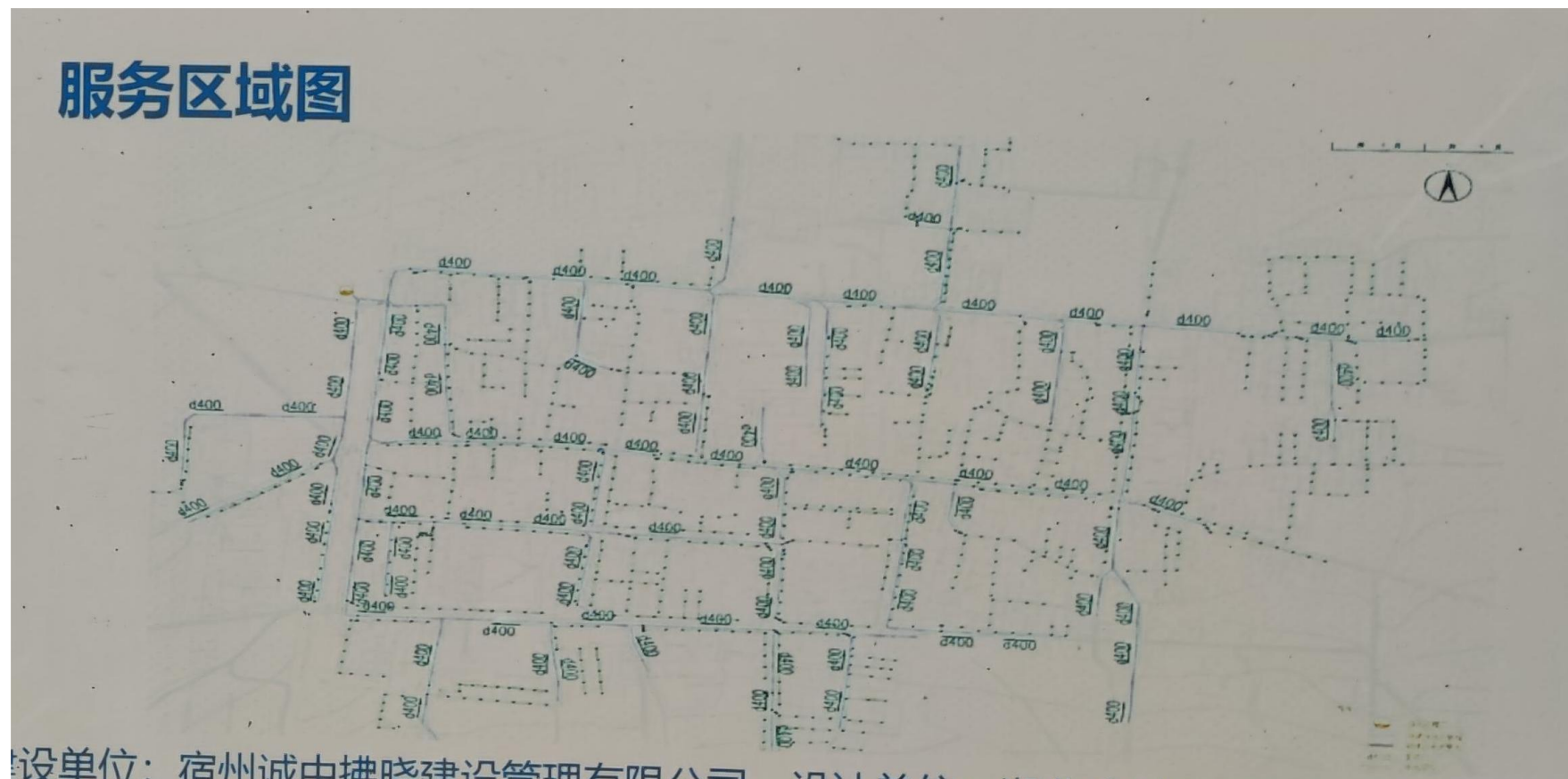
附图3 褚兰镇污水处理站污水收集管网分布图
